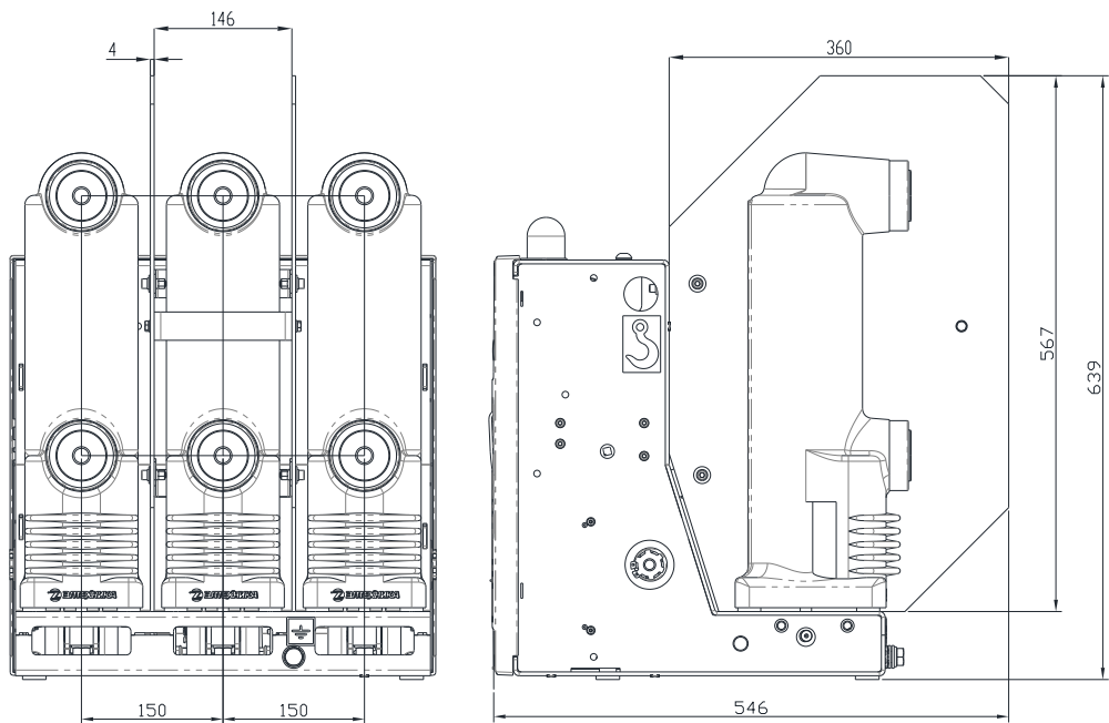
Рис. 1.3. Габаритно-присоединительные размеры выключателей в исполнении S с клеммным рядом.
