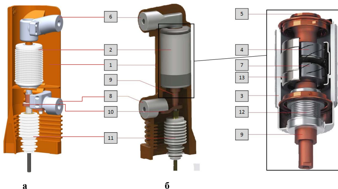
Рис. 2 Полус главной цепи (а - сборное исполнение, б - литое исполнение)
