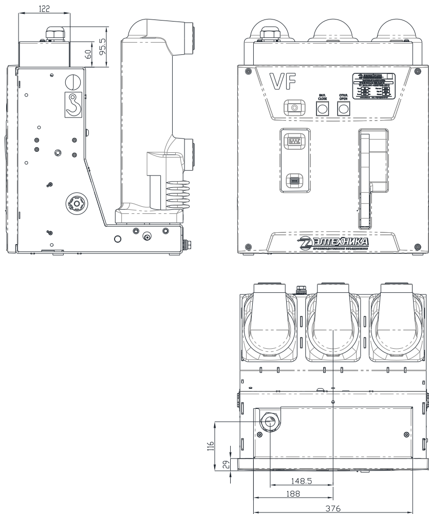
Рис. 1.3. Габаритно-присоединительные размеры выключателей в исполнении S с клеммным рядом.
