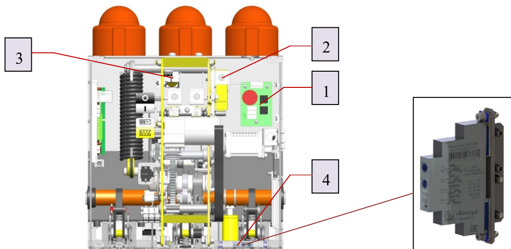
Рис. 10а Выключатель с опцией минимальный расцепитель напряжения:
