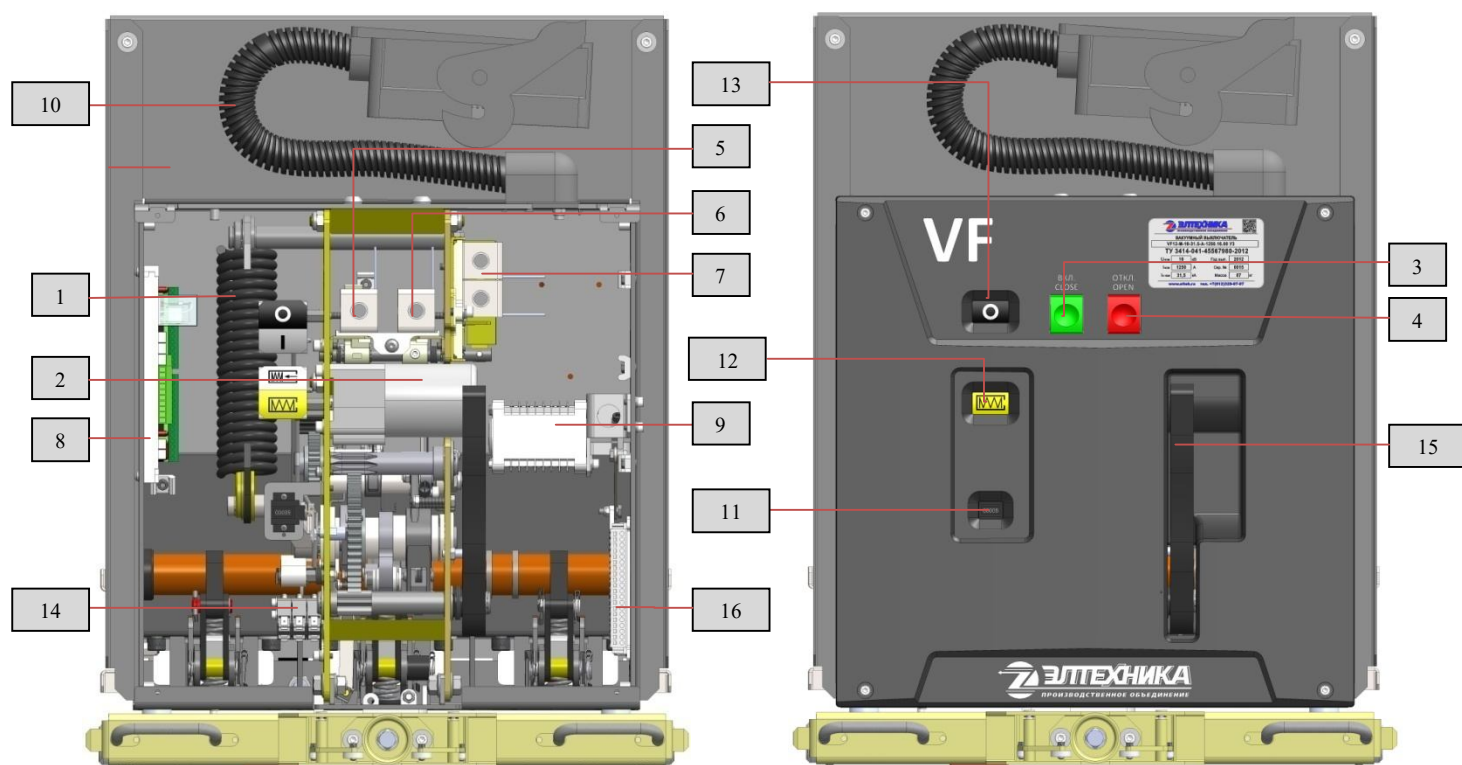
Рис. 3 Привод выключателя:
