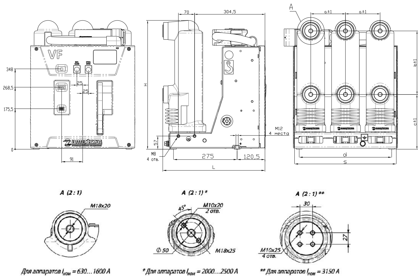
Рис. 1.1а Габаритно-присоединительные размеры выключателей в исполнении S без обрамления.
