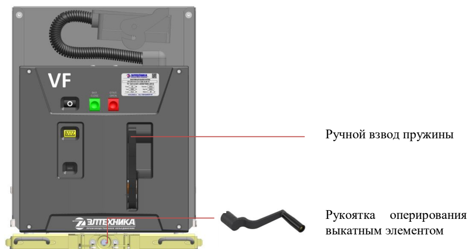
Рис. 13 Рукоятки
