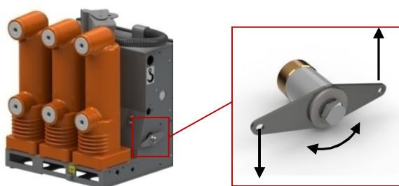
Рис. 8 Механическая блокировка внешних устройств
