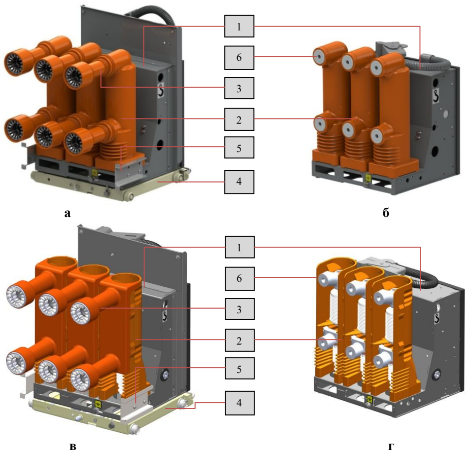
Рис. 1 Общий вид выключателей с корпусами полюсов в литом исполнении (а – исполнение М и Е, б – исполнение S) и сборном исполнении (в – исполнение М и Е, г – исполнение S): 1 – корпус с приводом; 2 – полюс главной цепи; 3 – токоведущие стержни с ламельными контактами; 4 – тележка аппаратная (тележка аппаратная моторизованная); 5 – планка управления шторочным механизмом; 6 – выводы полюсов главной цепи
