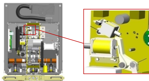
Рис. 9 Электромагнитная блокировка включения выключателя при отсутствии оперативного питания
