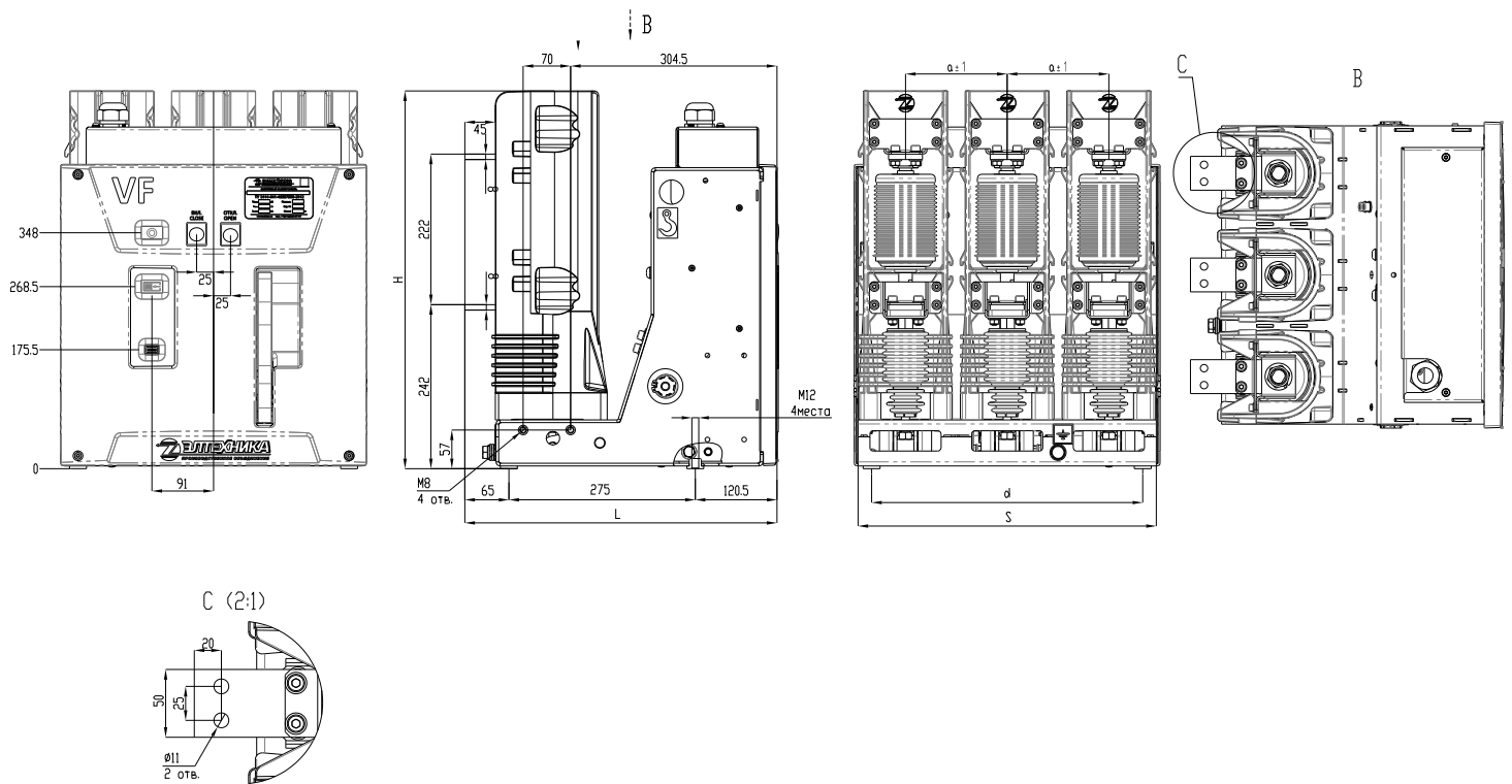
Рис. 1.16 Габаритно-присоединительные размеры выключателей в исполнении L.
