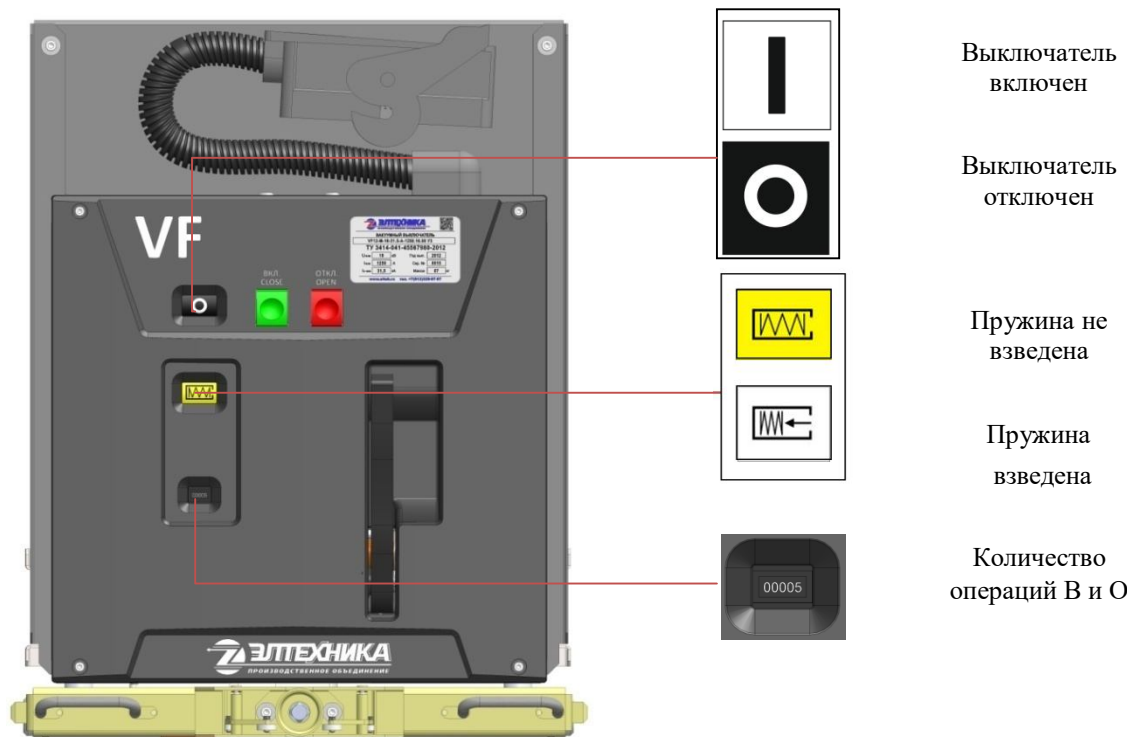
Рис. 4 Индикаторы на лицевой панели выключателя
