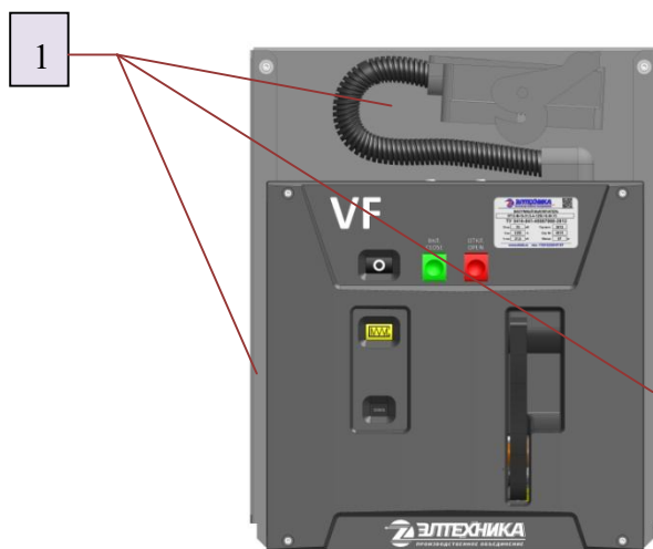
Рис. 12 Выключатель с опцией обрамление
