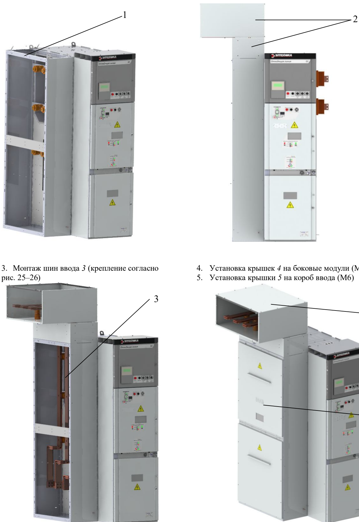
Рис. 31. Сборка шинного ввода сбоку шкафа КРУ
