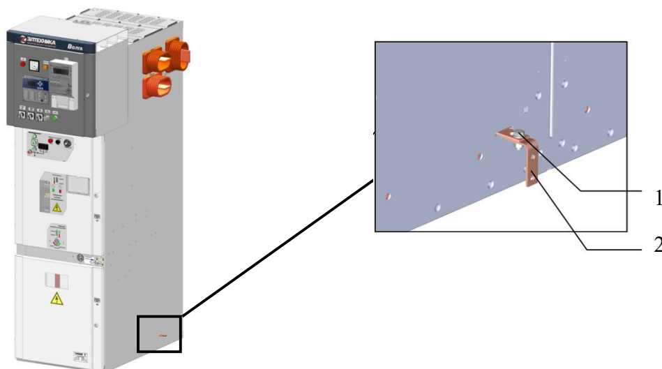
Рис. 23 Сборка системы заземления секции шкафов КРУ 1 – болтовое соединение М8; 2 – шина заземления соседнего шкафа КРУ
