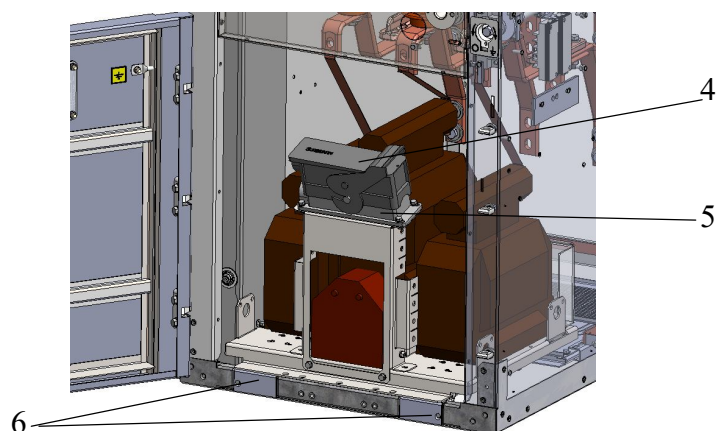
Рис. 286. Порядок монтажа выкатного элемента с измерительными трансформаторами напряжения в отсек кабельных соединений
