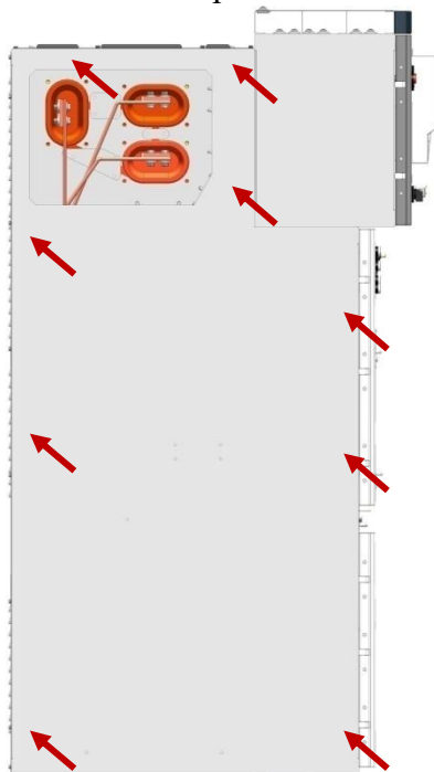
Рис. 22 Места скрепления соседних шкафов КРУ
