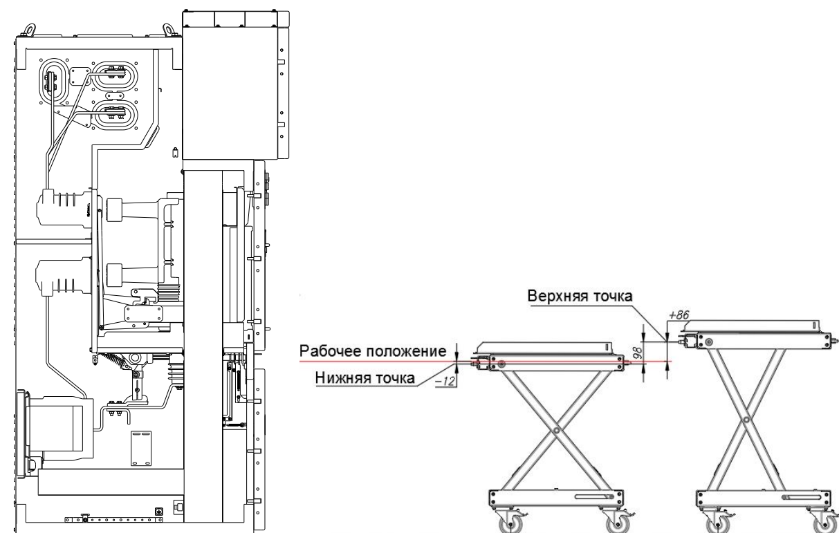
Рис. 10а Диапазон регулировки сервисной тележки по высоте
