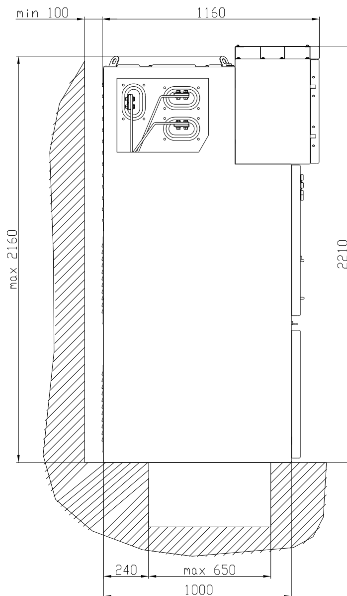
Рис. 2.3 Установка шкафов КРУ при одностороннем обслуживании
