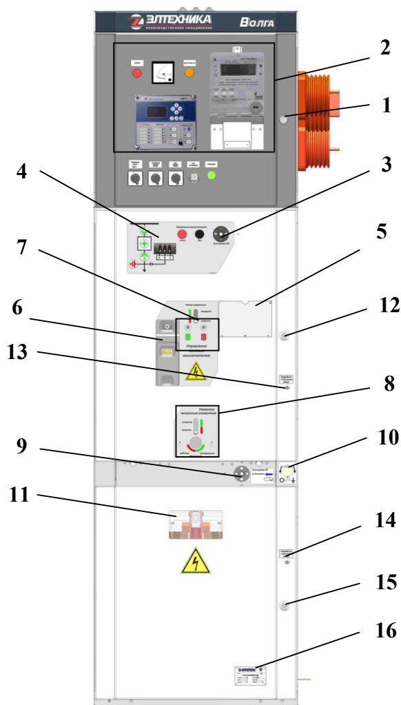
Рис. 2 Лицевая панель КРУ
