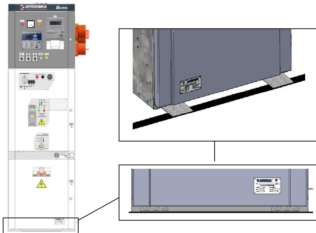
Рис. 24 Присоединение к внешнему контуру заземления
