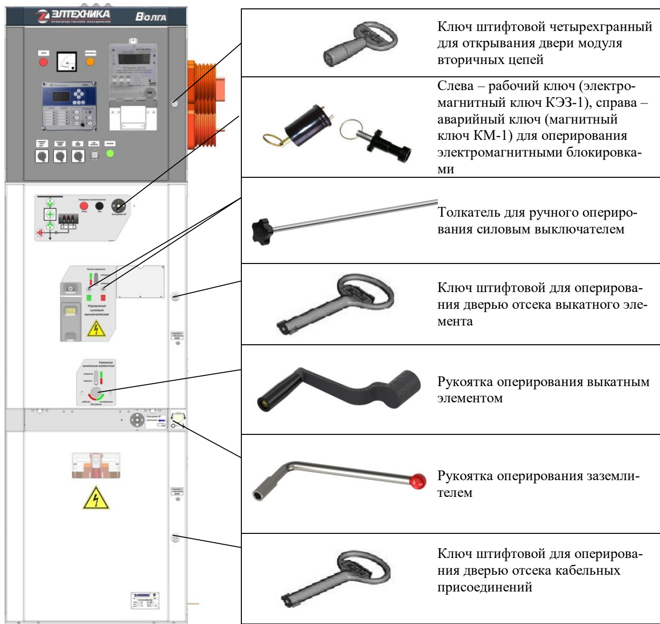
Рис. 3 Принадлежности шкафа КРУ
