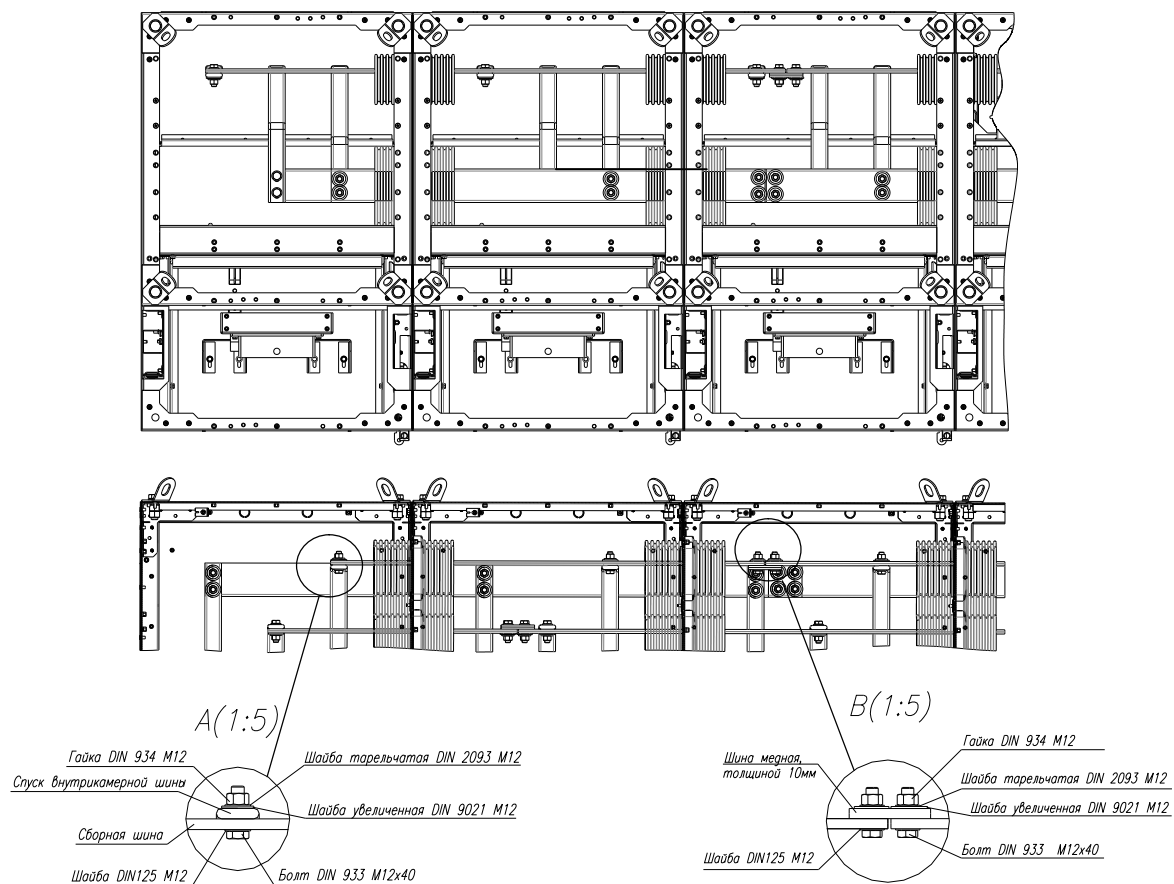
Рис. 26 Монтаж сборных шин (вид сверху на шкафы КРУ)
