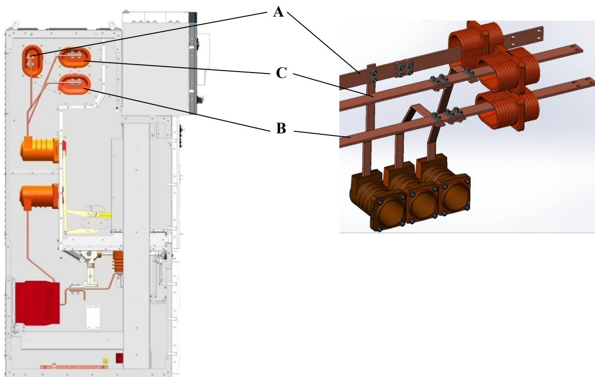
Рис. 25. Монтаж сборных шин
