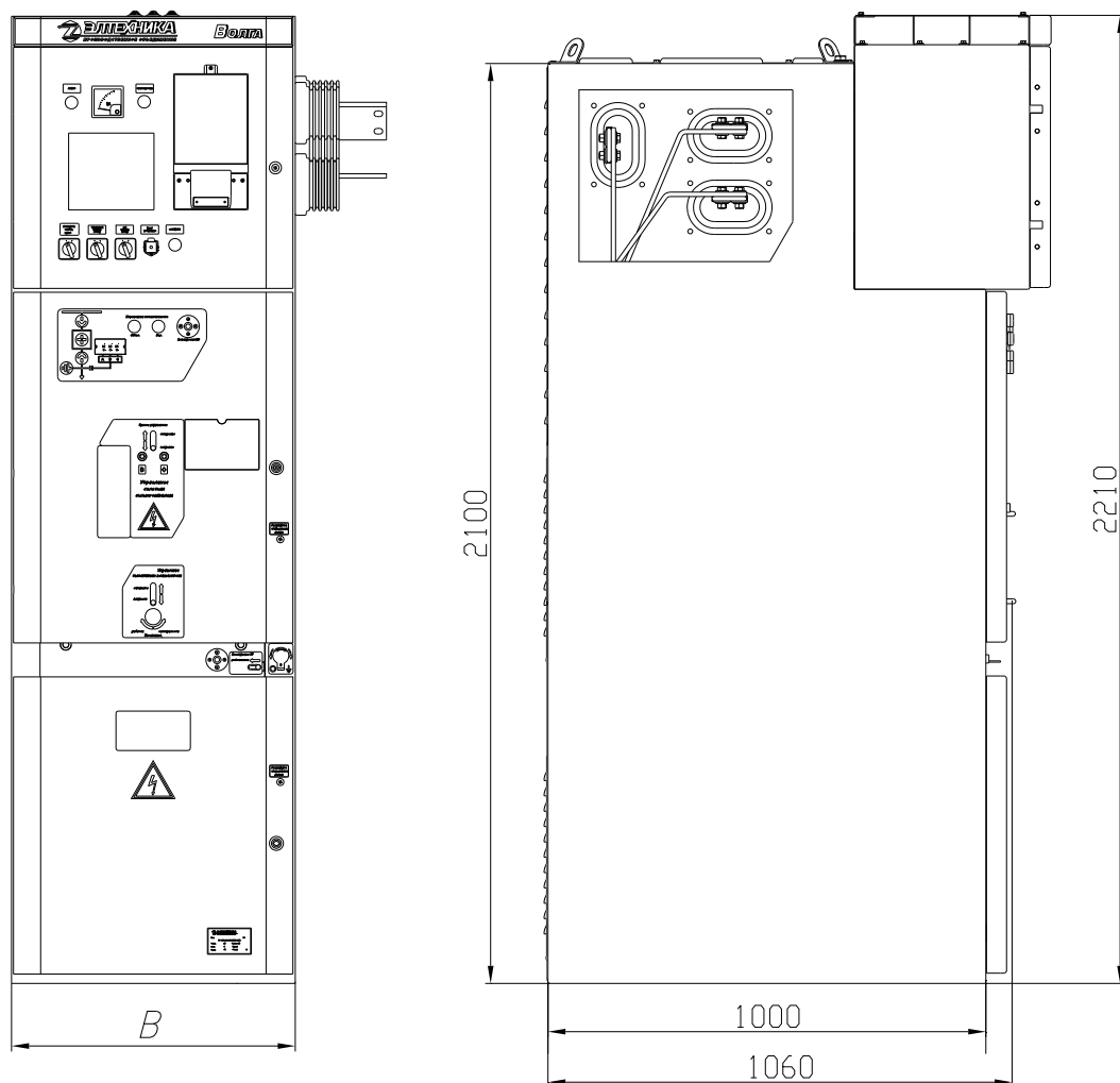
Рис. 2.1 Габаритные размеры шкафов КРУ
