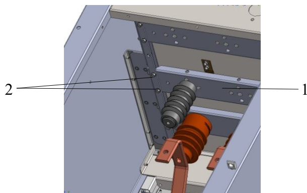
Рис. 33 Планка с ОПН
