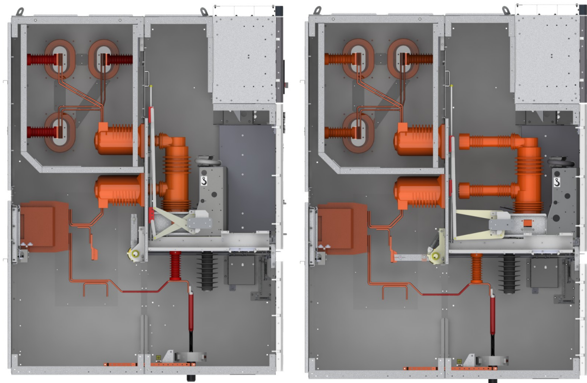
Рис. 7. Положения выкатных элементов на примере силового выключателя VF24 (слева – рабочее, справа – контрольное)
