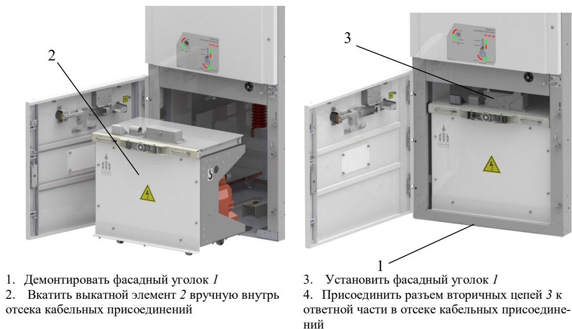
Рис. 32 Порядок монтажа выкатного элемента с измерительными трансформаторами напряжения в отсек кабельных присоединений
