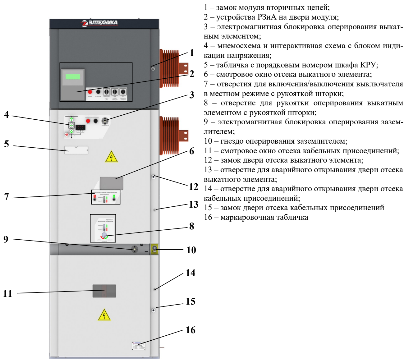
Рис. 2. Лицевая сторона КРУ
